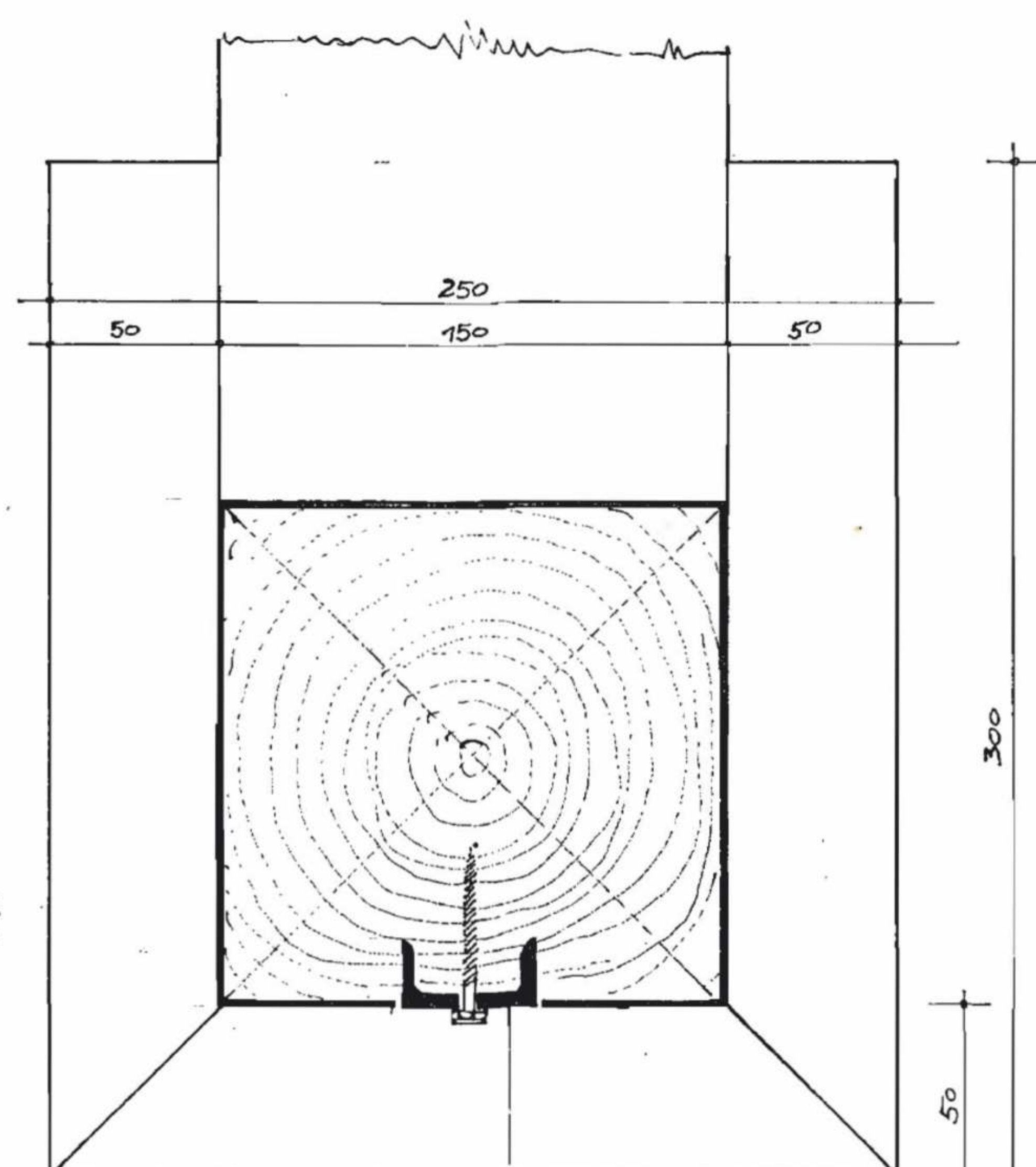
SCHNITT I M 1:20
